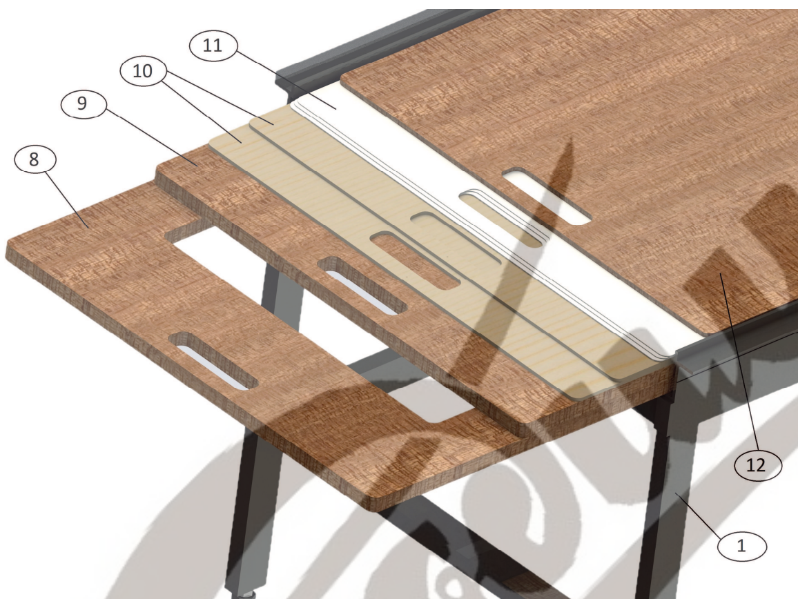
Рис.3 Компоновка подложек регулировки высоты пласта.
